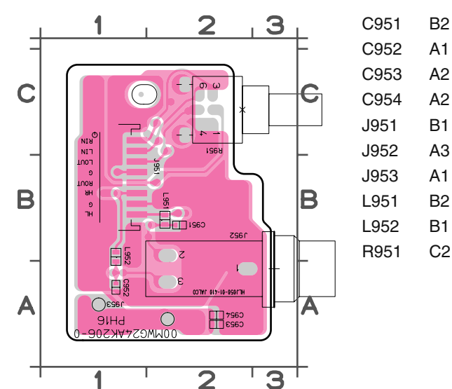
PH16 PCB
