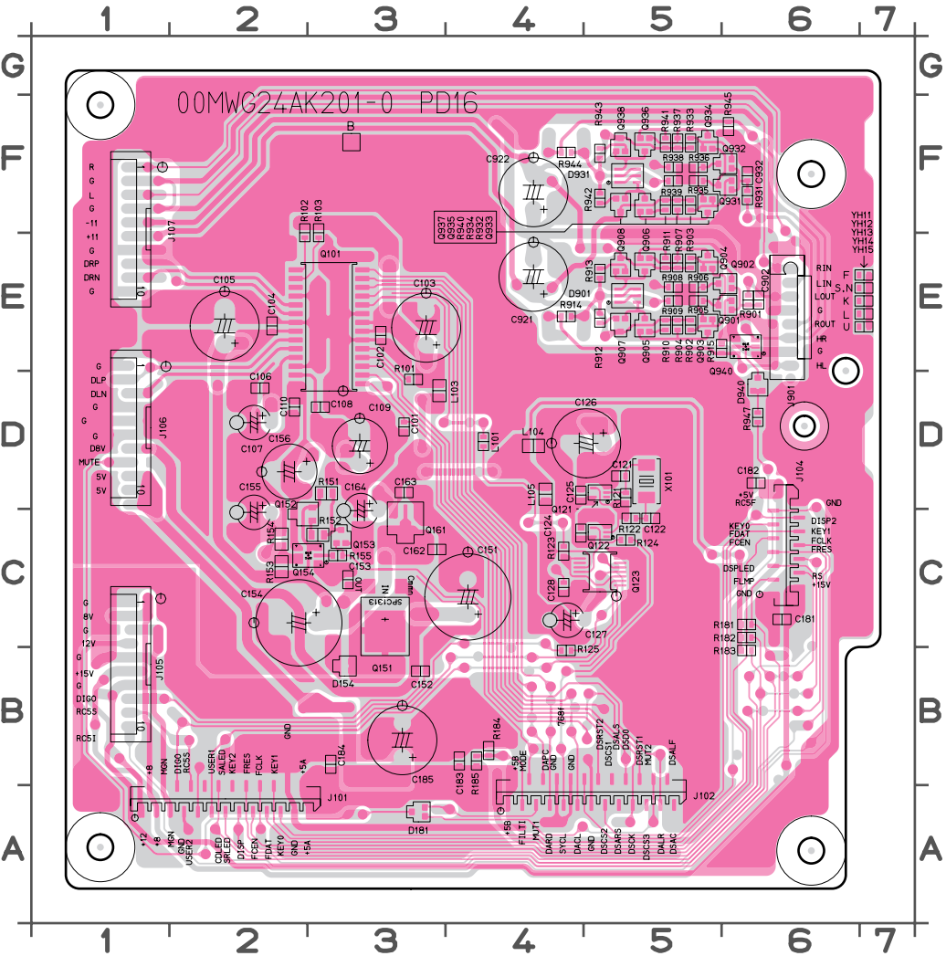
PD16 PCB
