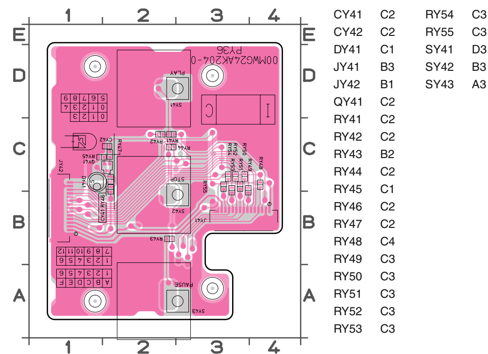
PY36 PCB
